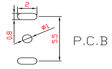
图为焊盘位置和大小
